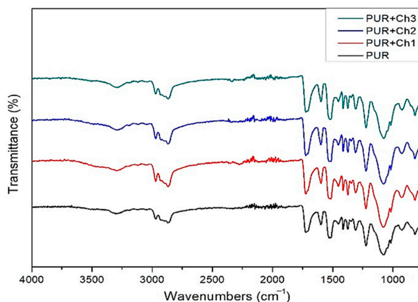
Figure 2. ATR-FTIR spectra.
