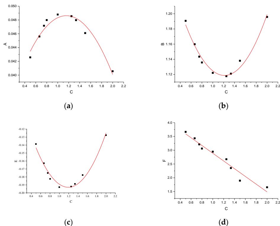
Figure 12. Parameter change curve with C. (a) Parameter A; (b) parameter B; (c) parameter C; (d) parameter D.
