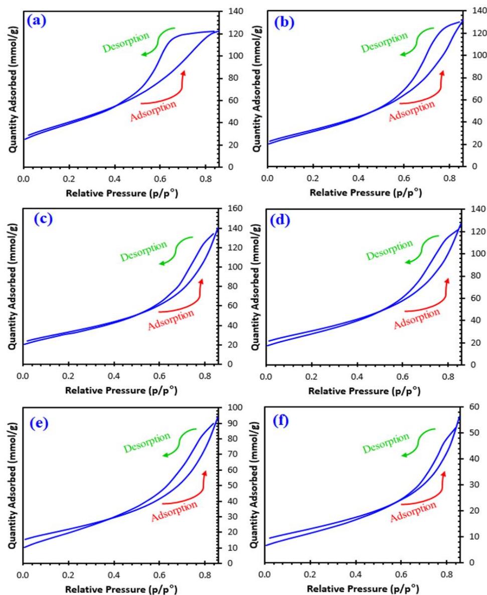
Figure 4. Nitrogen physisorption isotherm plots of; (a) x0, (b) x01, (c) x02, (d) x03, (e) x04, and (f) x05.
