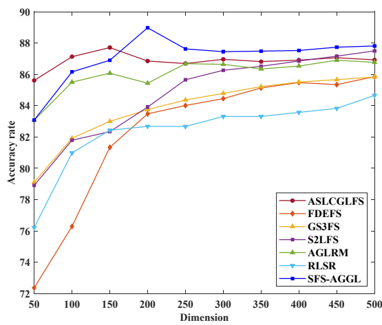
(b) CMU PIE
