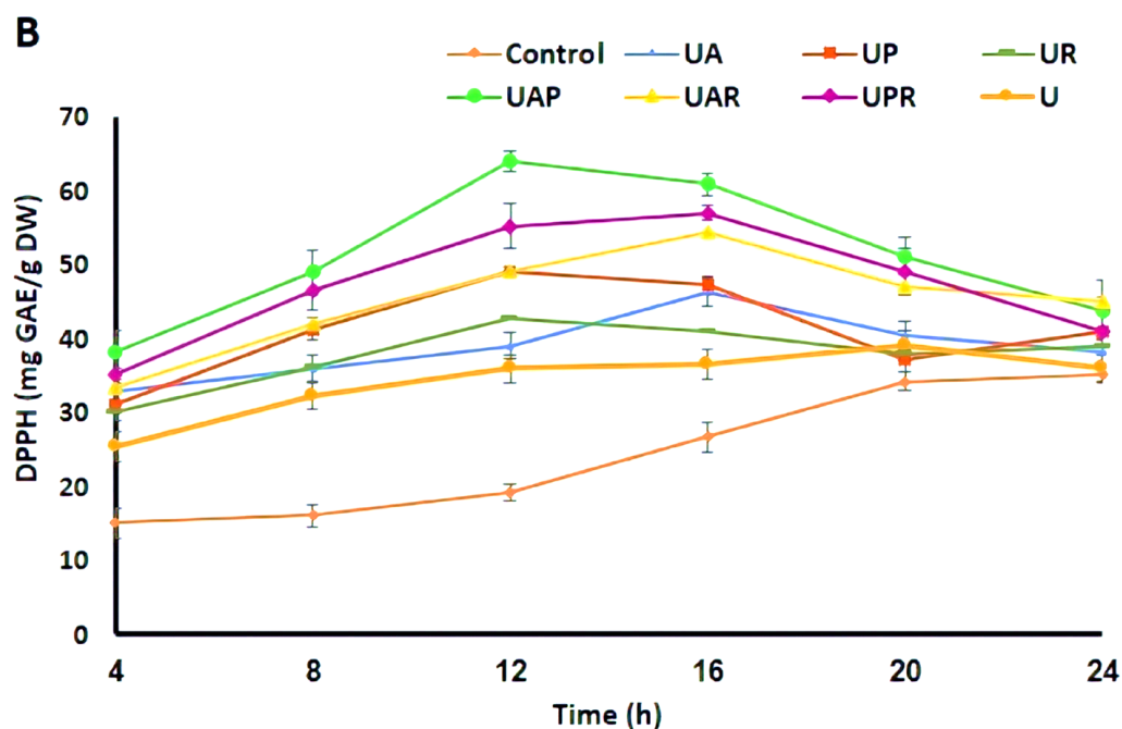
Figure 3. DPPH free radical scavenging activity of the (A) unfermented control, ultrasound-treated sample (U), and fermented E. amoenum using (A ( L. acidophilus ); P ( L. plantarum ); R ( L. reuteri ); AP ( L. acidophilus — L. plantarum ); AR ( L. acidophilus — L. reuteri ); PR ( L. plantarum — L. reuteri )); (B) unfermented control, ultrasound-treated sample (U), and ultrasound-assisted fermented E. amoenum (UA (Ultrasound-assisted L. acidophilus ); UP (Ultrasound-assisted L. plantarum ); UR (Ultrasound-assisted L. reuteri ); UAP (Ultrasound-assisted L. acidophilus — L. plantarum ); UAR (Ultrasound-assisted L. acidophilus — L. reuteri ); UPR (Ultrasound-assisted L. plantarum — L. reuteri )).
