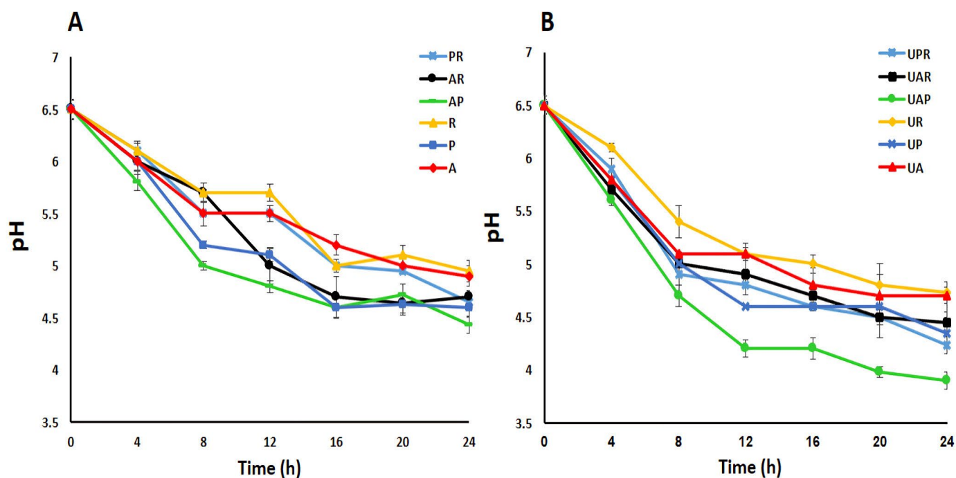
Figure 1. pH changes during the fermentation (A) and ultrasound-assisted fermentation (B) of E. amoenum . A ( L. acidophilus ); P ( L. plantarum ); R ( L. reuteri ); AP ( L. acidophilus — L. plantarum ); AR ( L. acidophilus — L. reuteri ); PR ( L. plantarum — L. reuteri ); UA (Ultrasound-assisted L. acidophilus ); UP (Ultrasound-assisted L. plantarum ); UR (Ultrasound-assisted L. reuteri ); UAP (Ultrasound-assisted L. acidophilus — L. plantarum ); UAR (Ultrasound-assisted L. acidophilus — L. reuteri ); UPR (Ultrasound-assisted L. plantarum — L. reuteri ).
