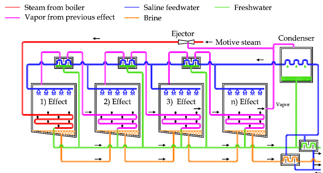
Figure 10. A schema of a TVC and MED unit.
