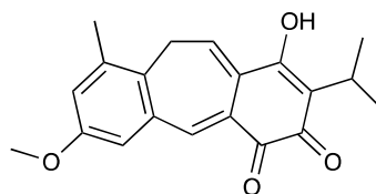
Fruticuline A (21)
