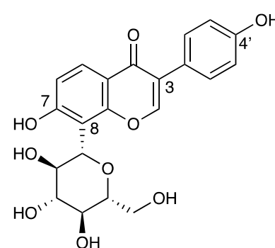
Puerarin (2)
