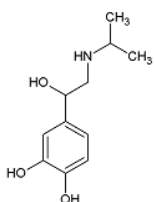
Isoproterenol
