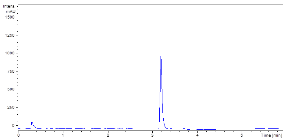
Compound 7e:
